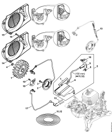
Система зажигания - Корпус вентилятора
