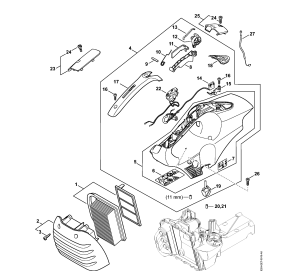
Воздушный фильтр - Кожух
