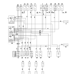
Схема контактов
