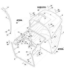
Травосборник
