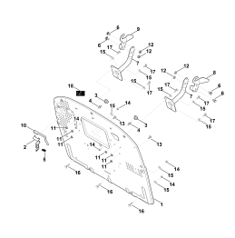
Задняя стенка
