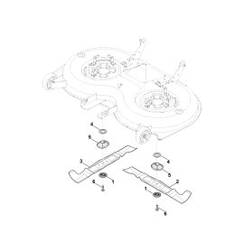
Нож
