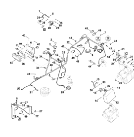
Узлы электрооборудования
