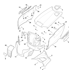
Кожух двигателя
