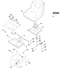
Сиденье
