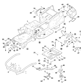
Рама
