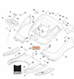
Кожух
