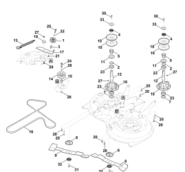
Привод ножа
