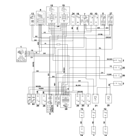
Схема контактов
