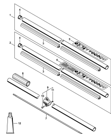
Хвостовик
