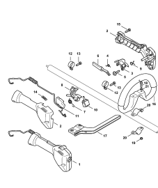
Рукоятка управления
