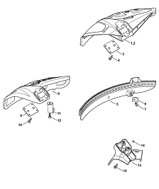
Защитное приспособление
